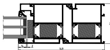
MB-70B Door – cross section
