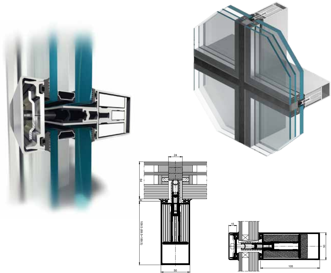
mullion – cross-section EI 45, EI 60
